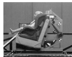
前面衝突試験
