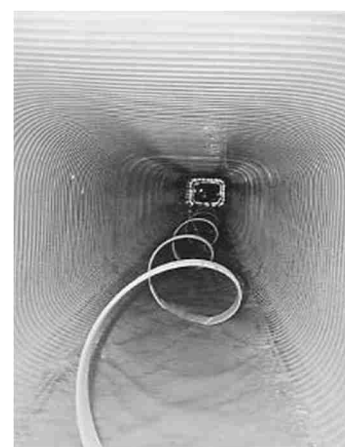
更生工法を施した管渠
