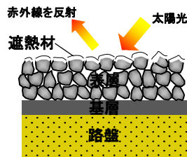
遮熱性舗装
