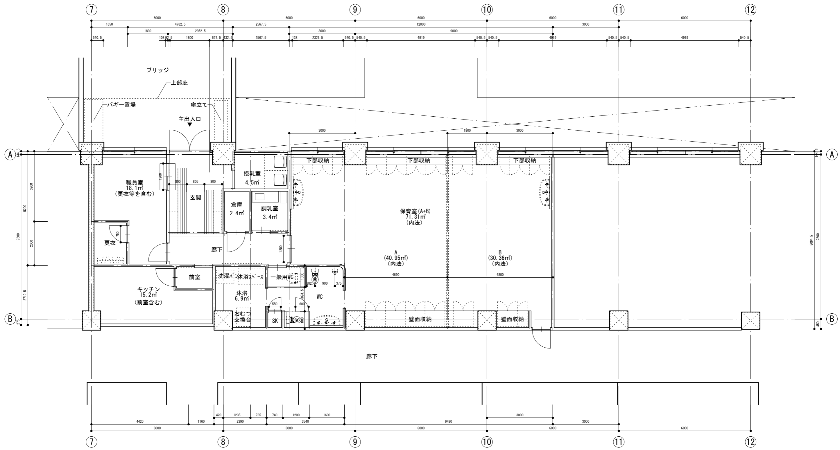
内閣府庁舎 保育所平面図
