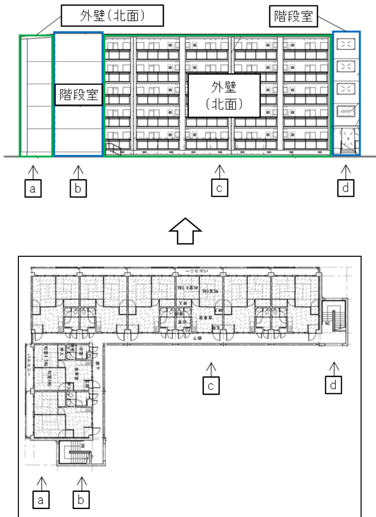
<外壁・階段室：L字型住棟の例>
