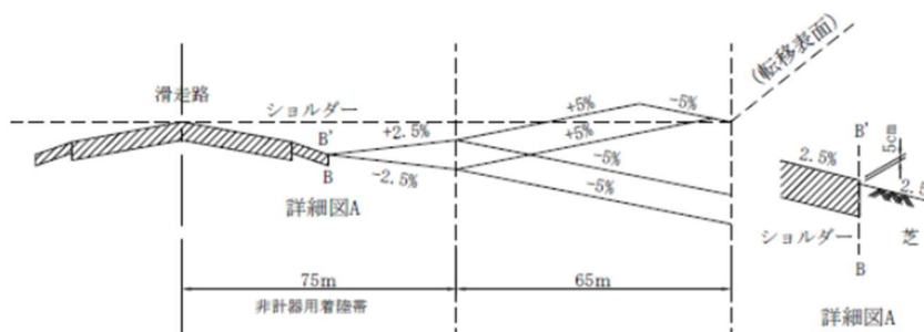
図-3.4.1 ショルダー（舗装）と着陸帯の植生部の境界 (コード番号 3 又は 4 の精密進入用滑走路の着陸帯の場合の例)
