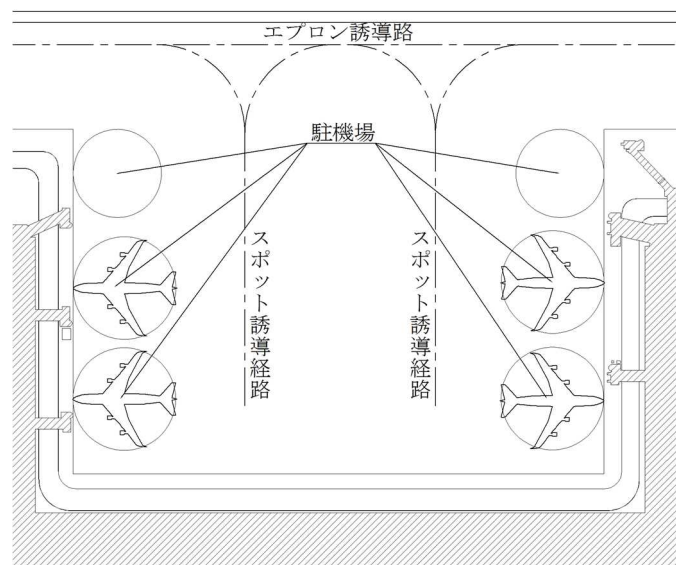
図-1.3 エプロン内の区分
