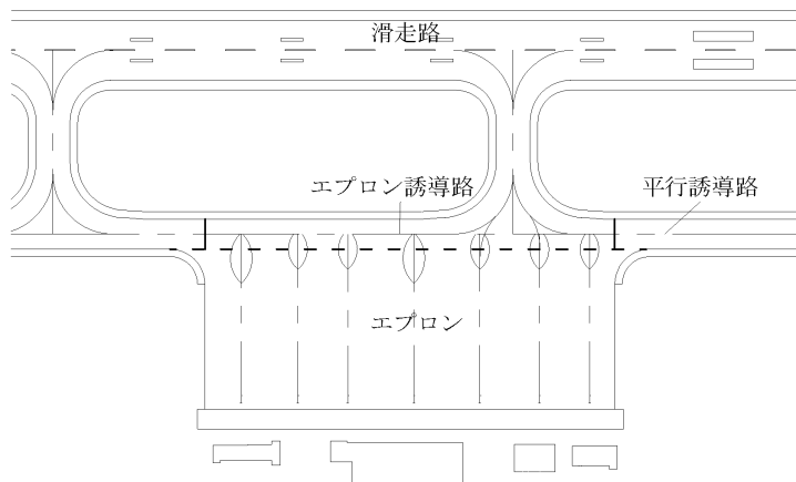
図-3.11.2 エプロン誘導路の例
