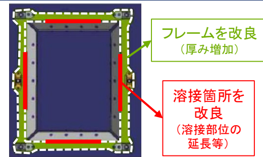
対策後のダクト取り付け部
