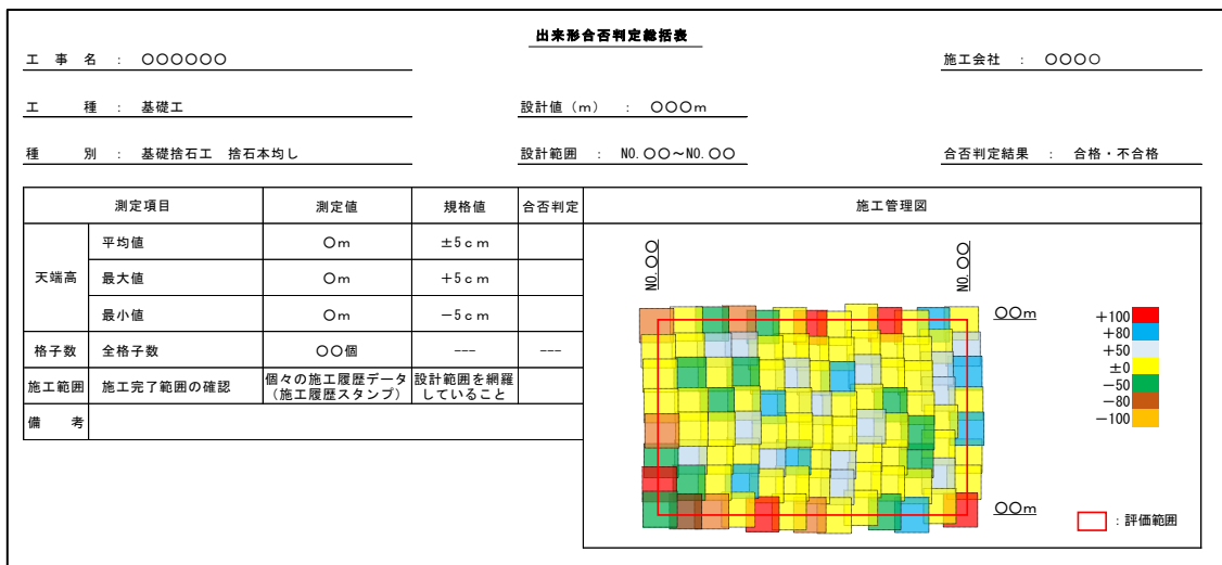
図- 2.2 出来形管理図表（本均し）（例）
