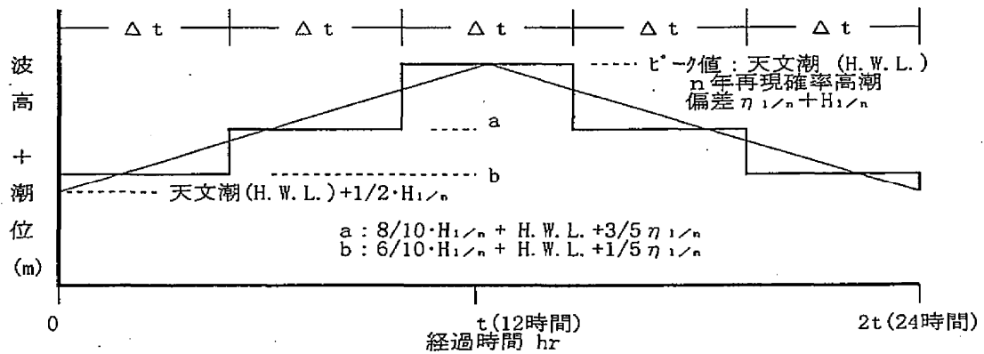
図V-7 波高と潮位を重ね合わせた時系列経過のモデル化(外洋に面する海岸の場合)
