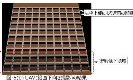
図-5(b) UAV(鉛直下向き撮影)の結果
