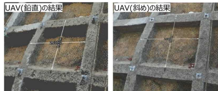
図-10 点群密度の比較
