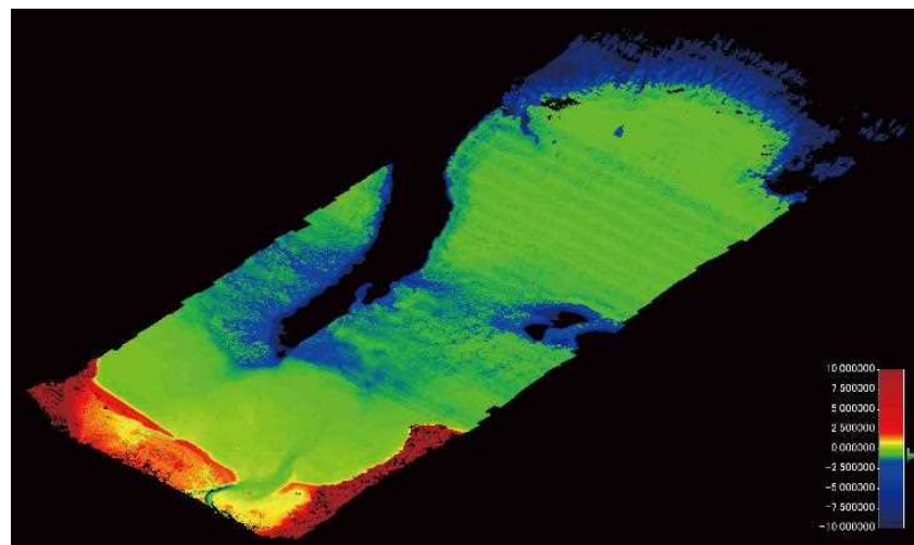
広範囲の複雑な地形を広範囲・高密度で測量
