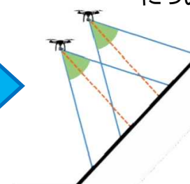
図-7 UAV斜め撮影
