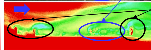
水制工周 辺の洗堀 標高(m)
